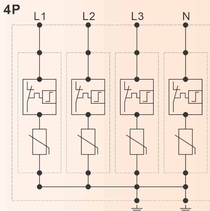
SPD-20-A280/4P
