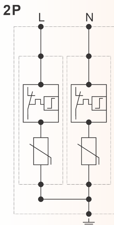
SPD-20-A280/2P
